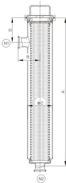
管式过滤器 Tube filter
